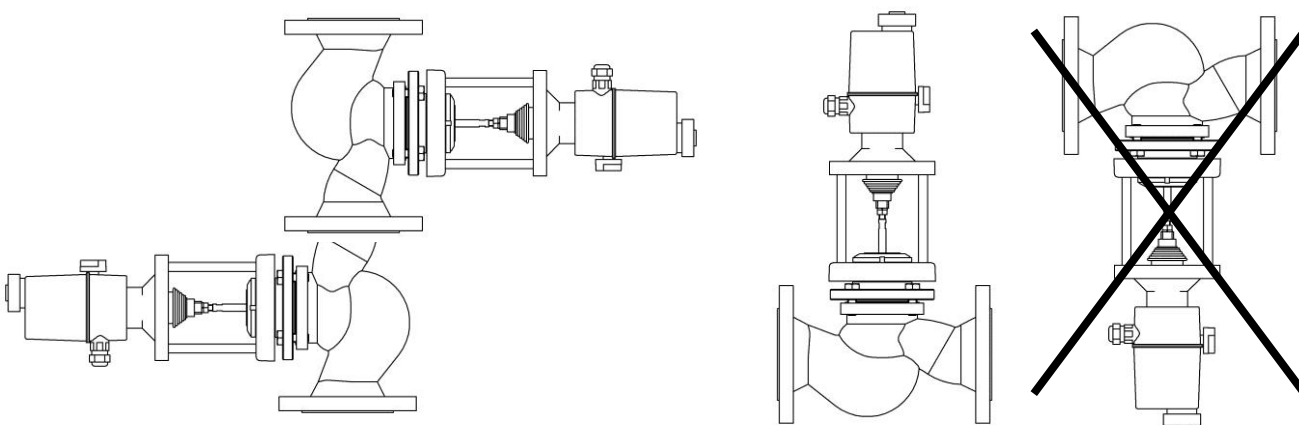
Рисунок А.5 Монтажные положения клапана с приводами REGADA ST 0; SAUTER AVF 234S F232.
