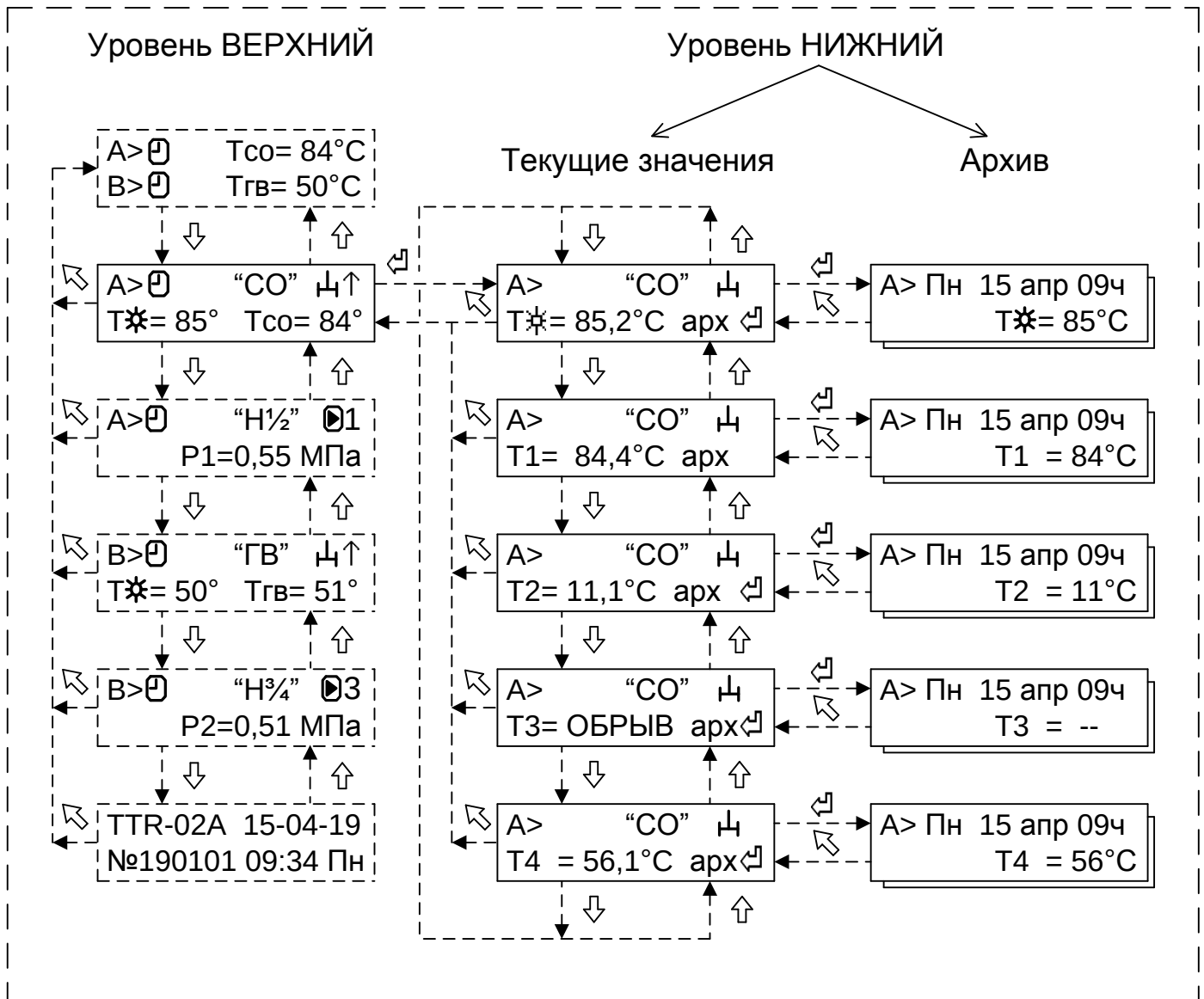
Рисунок 3 – Структура меню просмотра текущих и архивных значений температур
